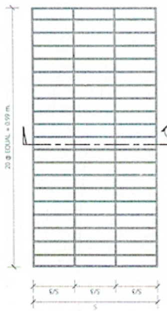
แปลนฝาเปิดทรง (G = 0.40 - 0.50) 1 : 10
