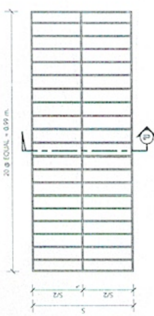
แปลนฝาเปิดทรง (G = 0.20 - 0.30) 1 : 10
